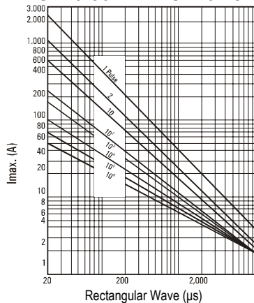
ROV10-561K – ROV10-182K
