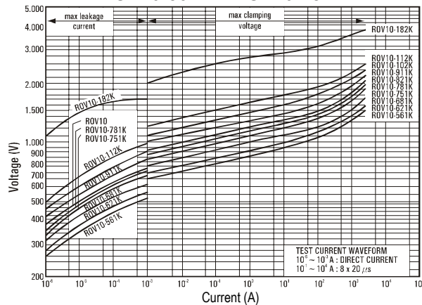
ROV10-561K – ROV10-182K
