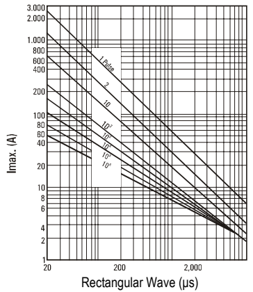
ROV10-561K – ROV10-182K
