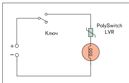
Рис. 7. Стандартная схема применения устройства PolySwitch в цепи мотора
