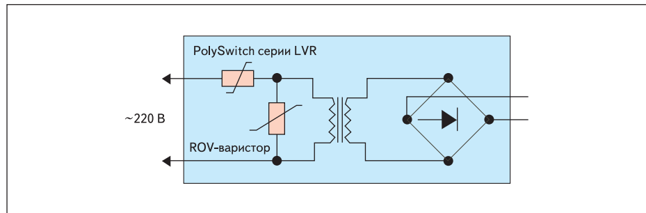
Рис. 8. Согласованная защита по току и напряжению в цепи сетевого напряжения
