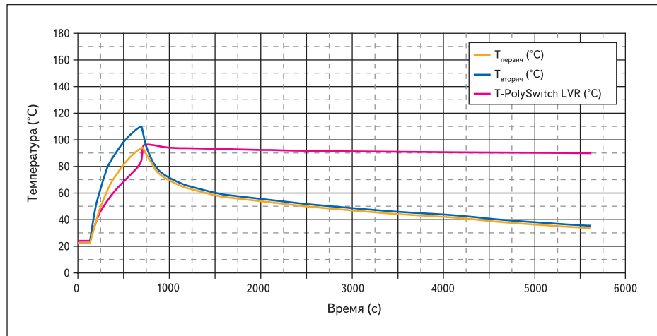
Рис. 2. Короткое замыкание во вторичной цепи трансформатора ~240 В, использующего PolySwitch серии LVR в качестве элемента первичной защиты
