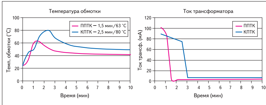
Рис. 3. Сравнение устройств КПТК и ППТК в случае короткого замыкания во вторичной цепи трансформатора ~120 В
